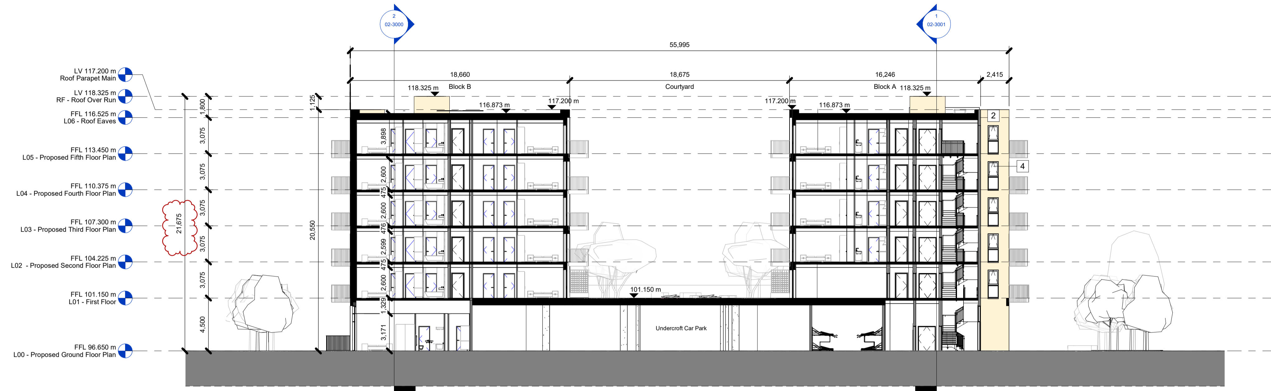
GA Section AA 1 : 200
