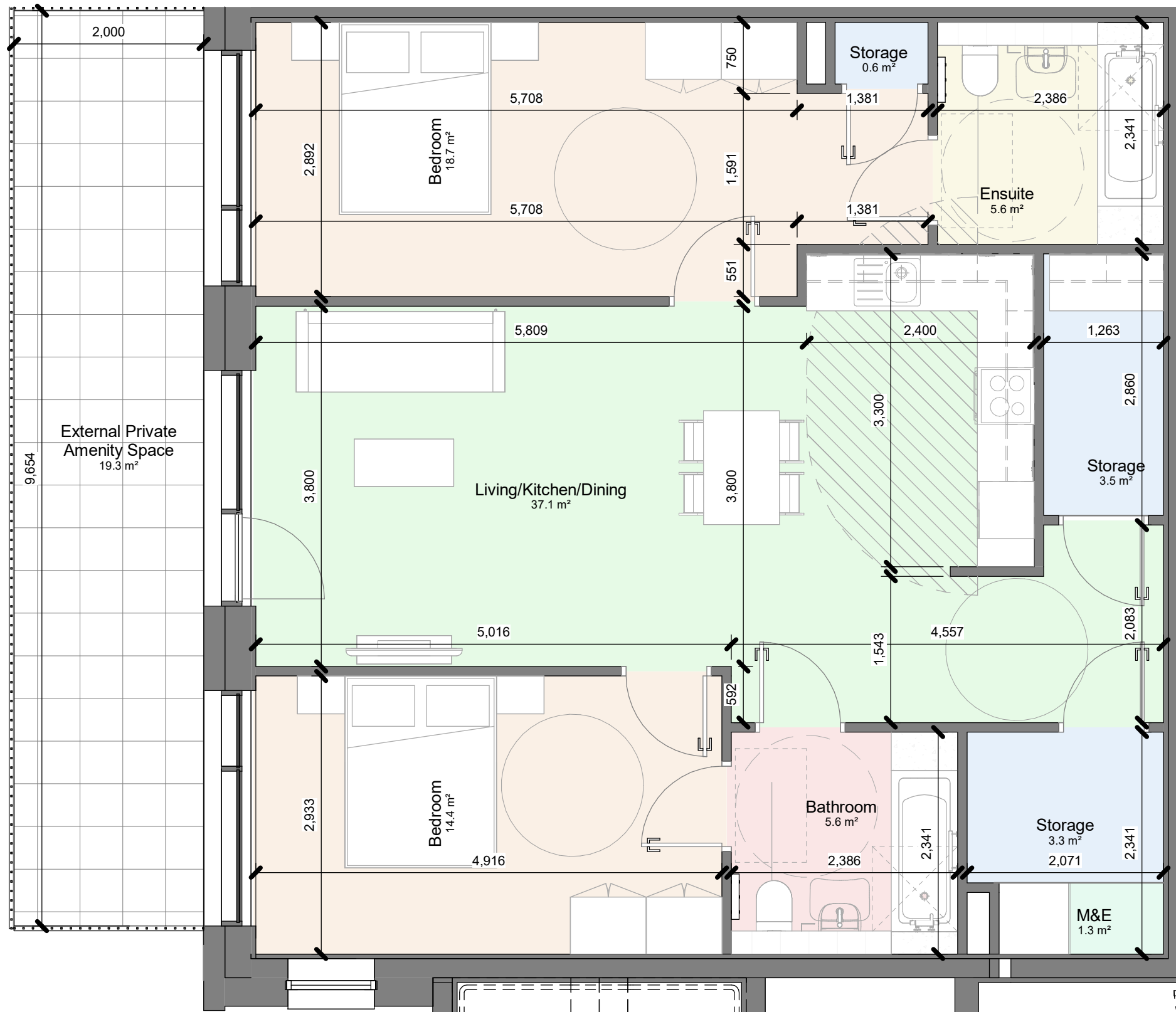
Apt Type 02 UD - 2B4P 1 : 50
